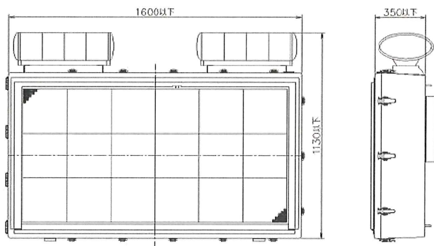
参考図 図1 車載式標識装置 (C) 外形図
