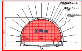
トンネル断面図 CII
