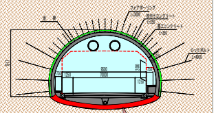
インパート
